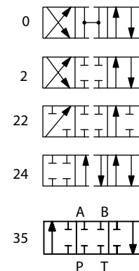
DG4V-3(S)-*BLV
