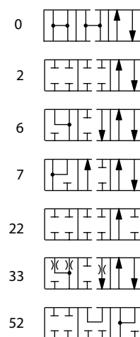
DG4V-3(S)-*BLV
