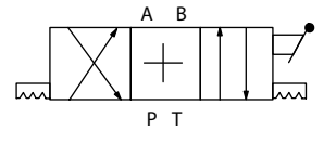
DG17V4-01*NL-10
