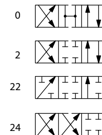
DG4V-3(S)-*ALV
