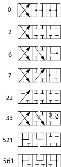
DG4V-3(S)-*BV
