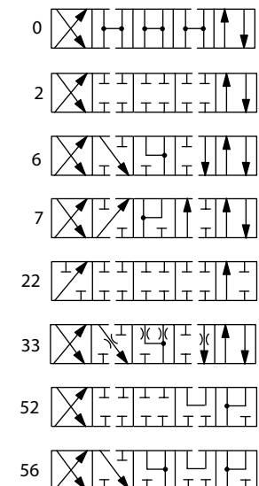
DG4V-3(S)-*CV
