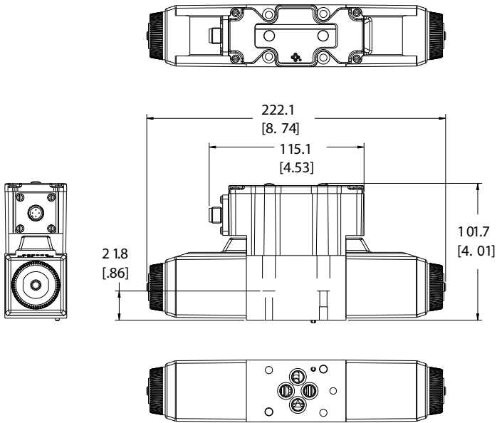
DG4V-3-*C/N-*M-PM4*S-***7-70
